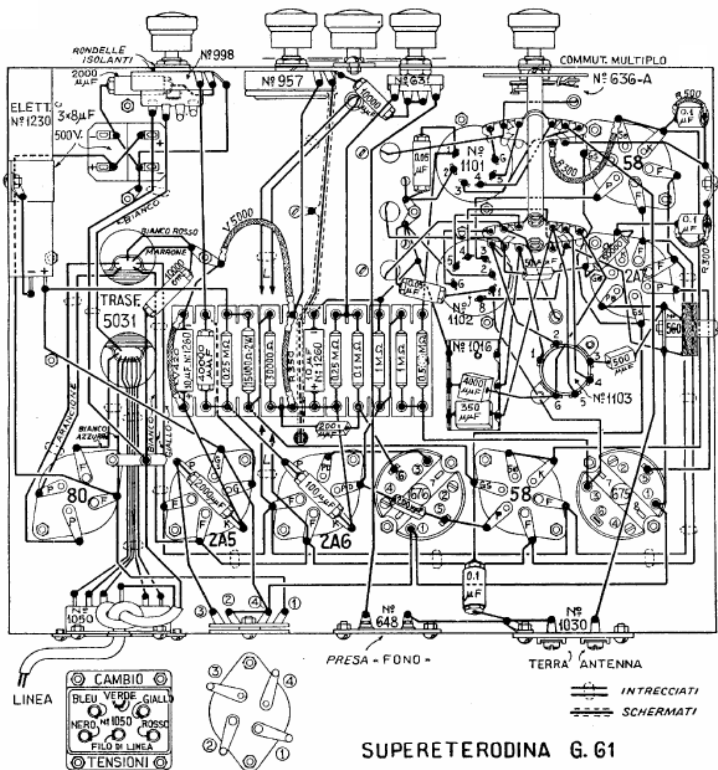
Schema costruttivo della Super G-61.
